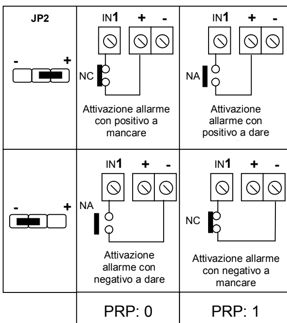
Modalità del segnale per il comando di allarme degli ingressi
