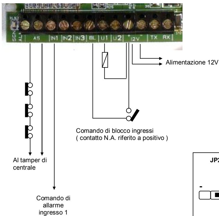
Modalità del segnale per il comando di allarme degli ingressi
